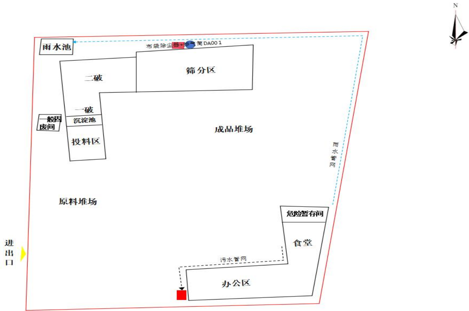
附图3 项目总平面布置图及雨污管网图
