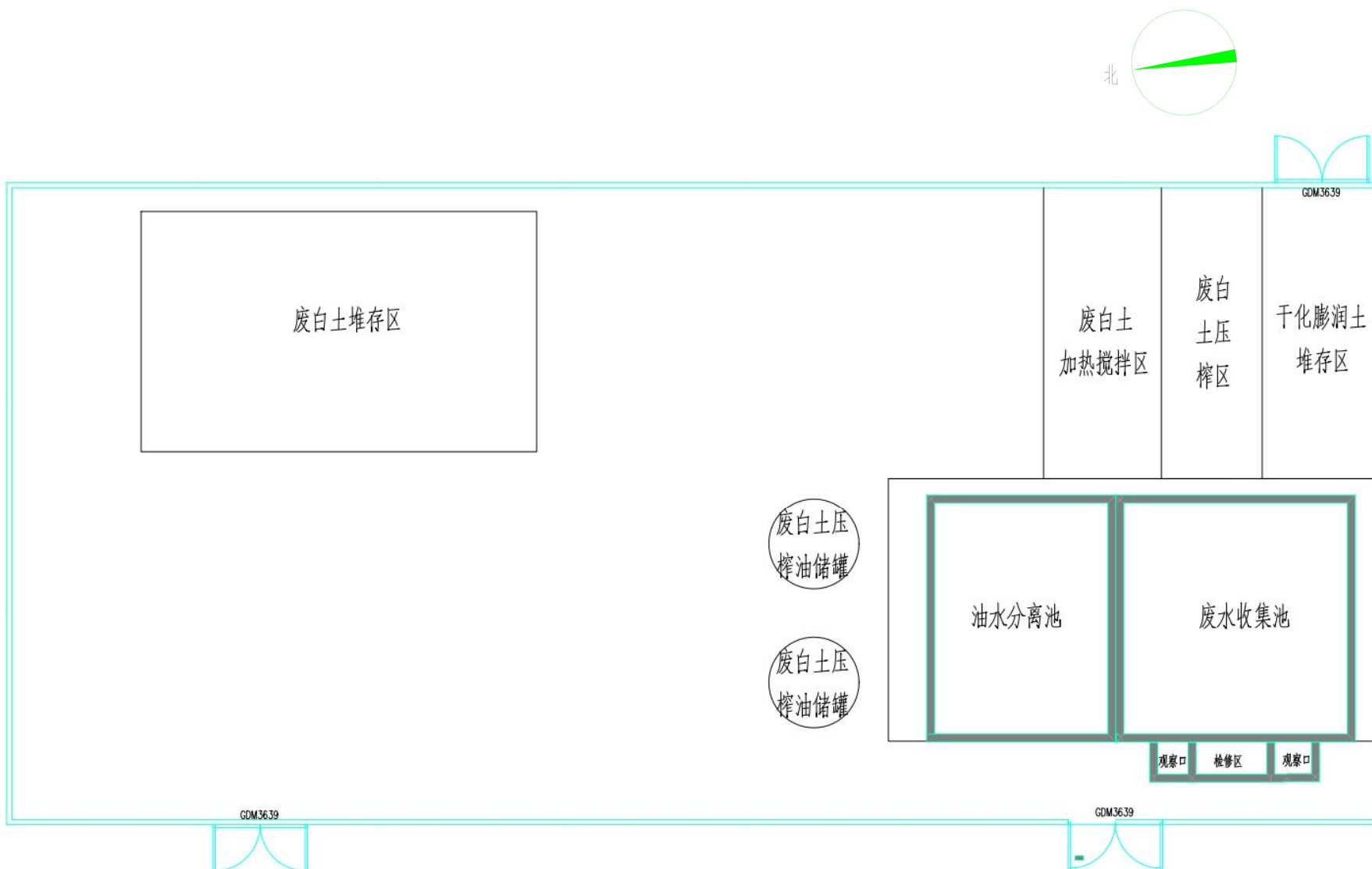
附图 6 项目废白土压榨车间平面布置图
