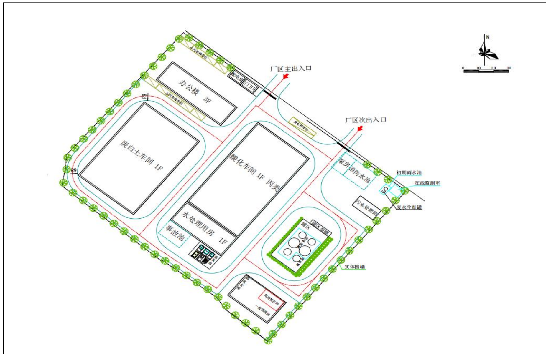
附图 4 项目厂区总平面布置图
