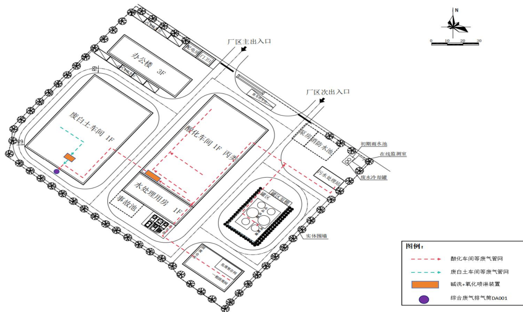
附图 8 项目厂区废气管网及环保设施分布图
